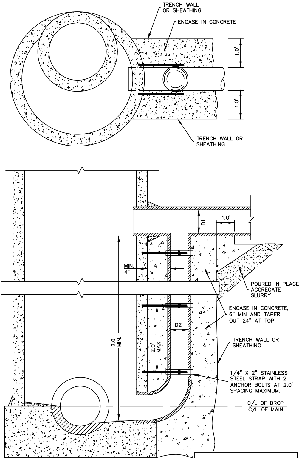
OUTSIDE DROP MANHOLE N.T.S.
