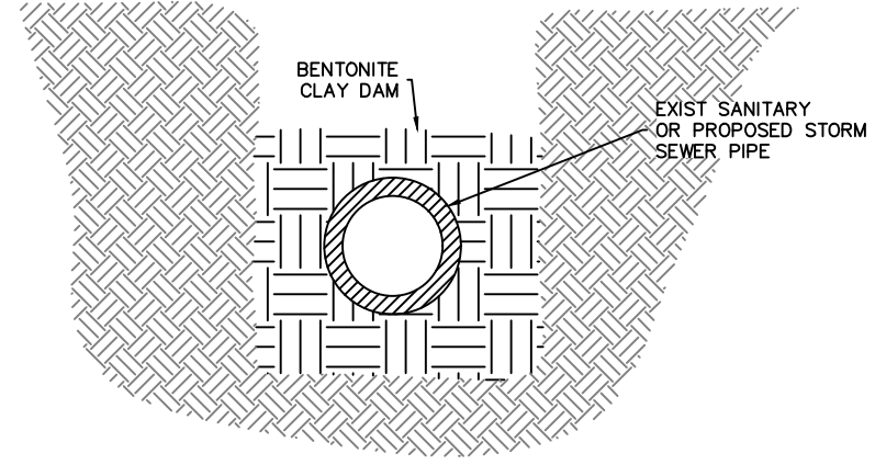
BENTONITE CLAY DAM DETAIL N.T.S.
